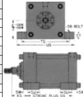
Side Lug Model 72-B (NFPA MS2)
