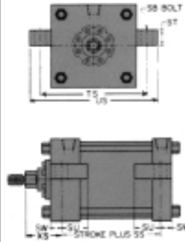
Centerline Lug Model 73-B (NPPA MS3)
